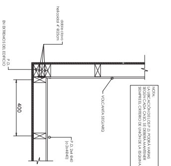
Detalle union encuentro muros ESCALA 1:10
