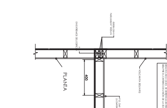
Detalle unión encuentro muros ESCALA 1:10
