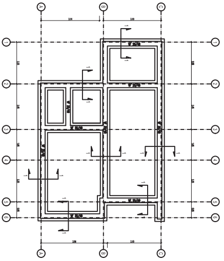
VIVIENDA CONTINUA - PLANTA FUNDACIONES ESCALA 1:50
