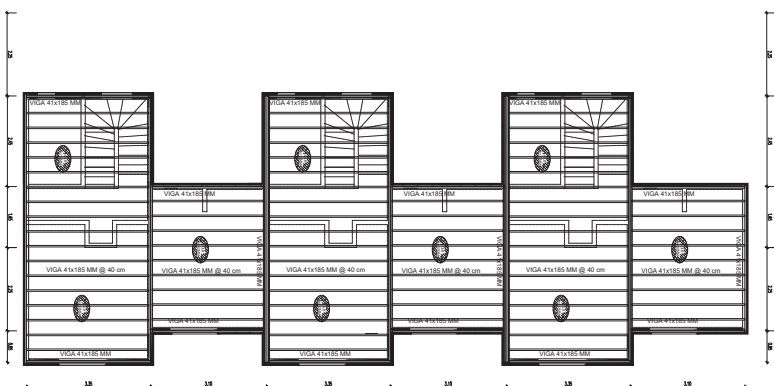
Planta Estructura de Cubierta Nivel +5.40 ESCALA 1:50
