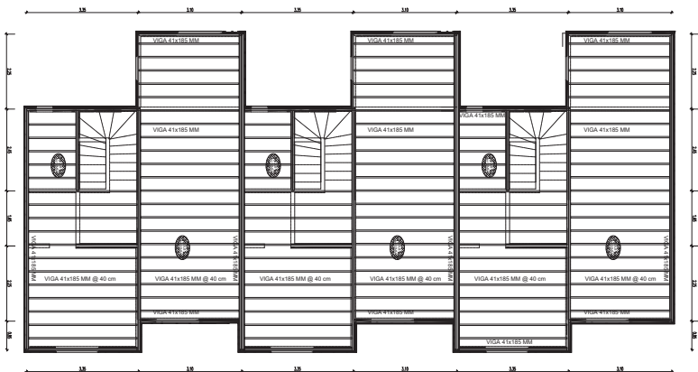
Planta Estructura de Entrepiso Nivel +2.60 ESCALA 1:50
