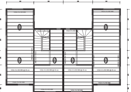
Planta Estructura de Entrepiso Nivel +2.60 ESCALA 1:50
