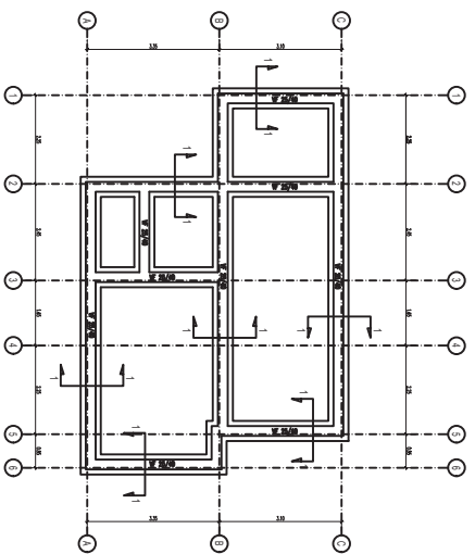
VIVIENDA PAREDADA - PLANTA FUNDACIONES ESCALA 1:50
