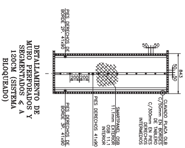
Detalle Entrepiso con Solera (Muro Medianero) - Nivel de Hold-down ESCALA 1:20
