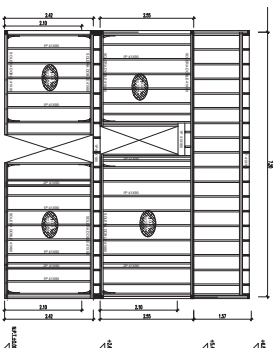
Elevación Estructural EIE B - EIE D - EIE F ESCALA 1:50
