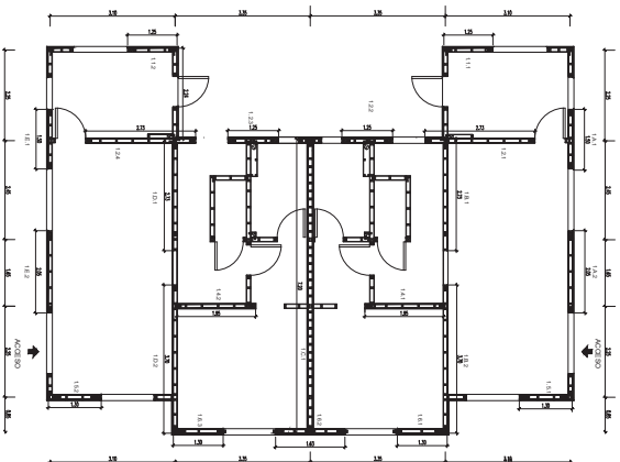
Planta Estructural Piso 1 Nivel 0.00 ESCALA 1:50
