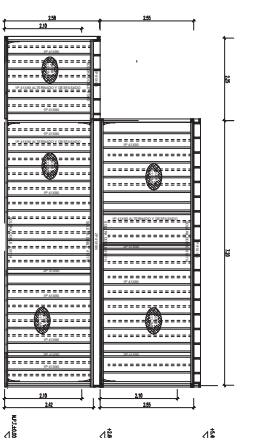
Elevación Estructural EIE C - EIE E ESCALA 1:50
