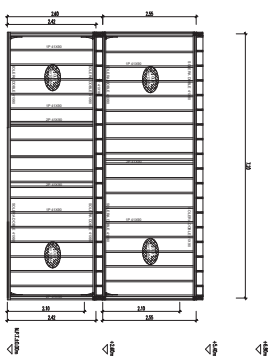
Elevación Estructural EIE C ESCALA 1:50
