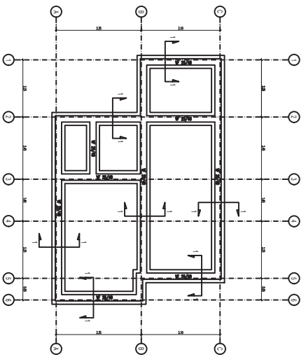
VIVIENDA ASLADA - PLANTA FUNDACIONES ESCALA 1:50
