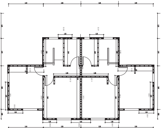
Planta Estructural Piso 2 Nivel +2.60 ESCALA 1:50
