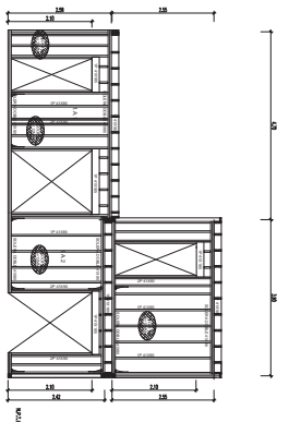
Elevación Estructural EIE A - EIE E ESCALA 1:50
