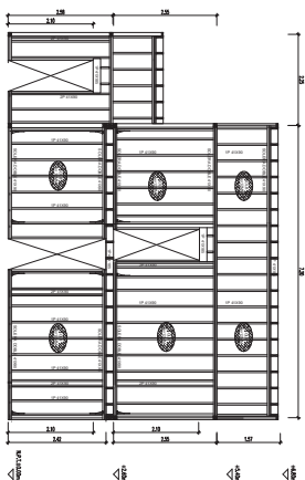
Elevación Estructural EIE B - EIE D ESCALA 1:50
