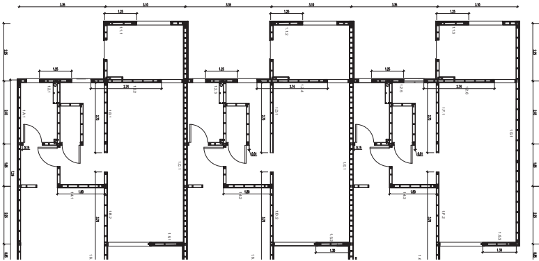
Planta Estructura Piso 1 Nivel 0.00 ESCALA 1:50
