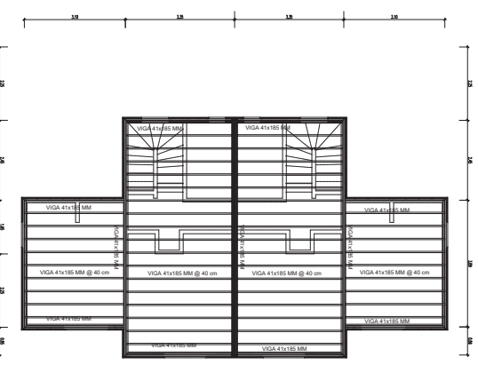
Planta Estructura de Cubierta Nivel +5.40 ESCALA 1:50
