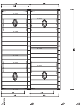
Elevación Estructural EIE A ESCALA 1:50
