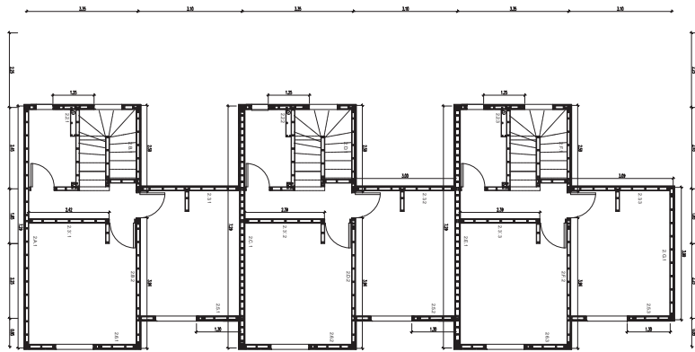
Planta Estructura Piso 2 Nivel +2.60 ESCALA 1:50
